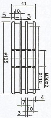
PISTON
