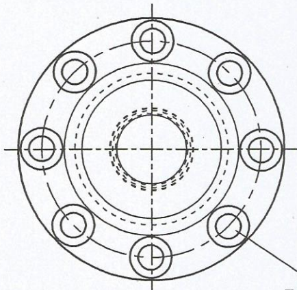
GLAND
