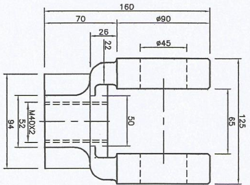
YOKE
