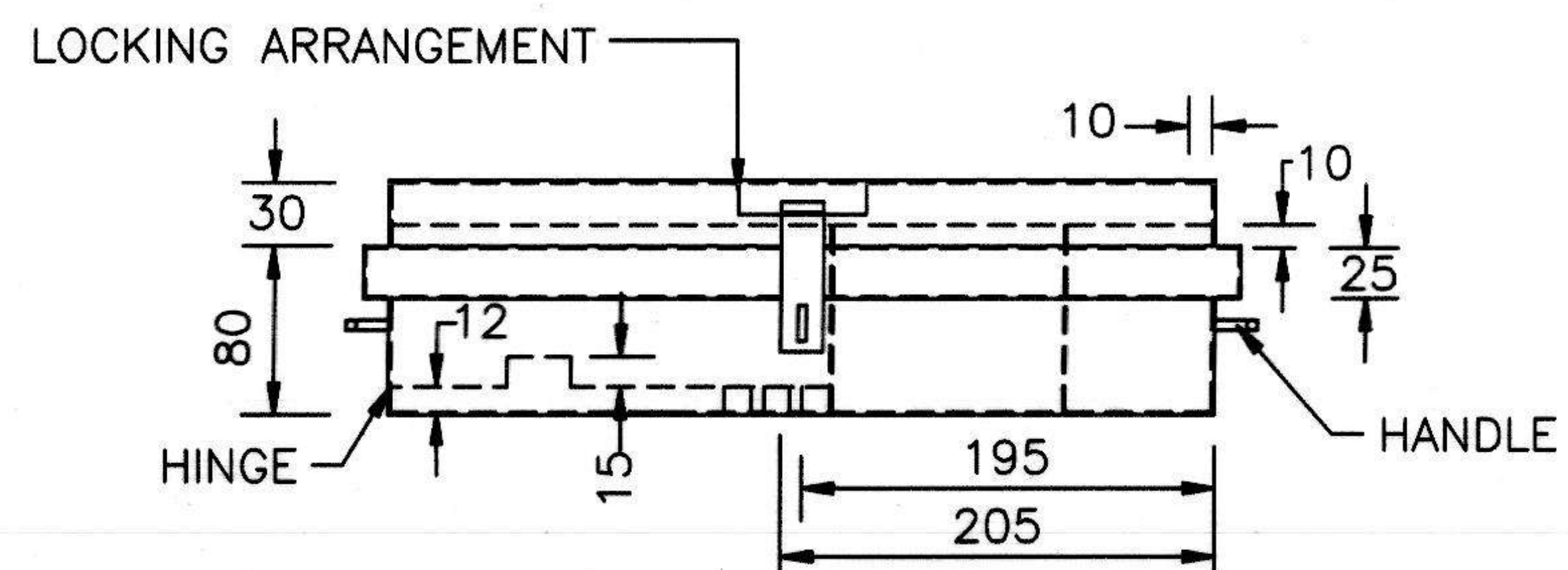
ELEVATION
