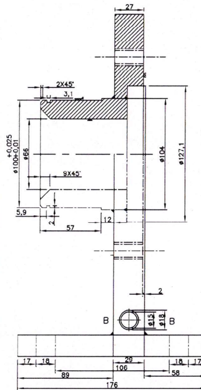
SEC A-A
