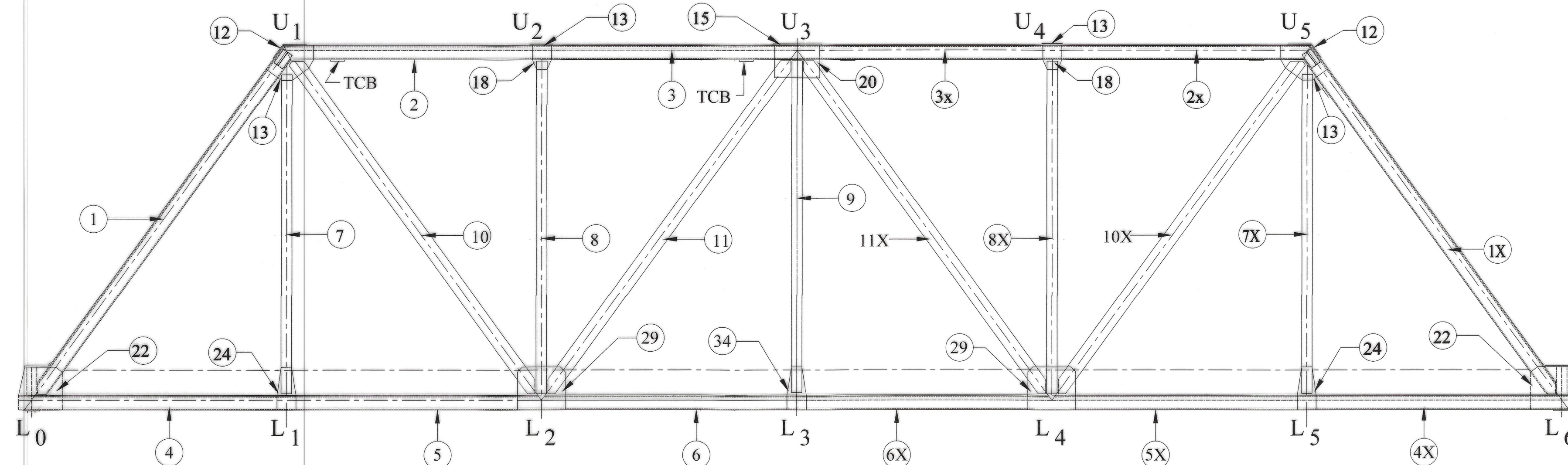
ELEVATION
